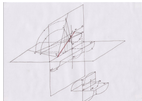
Géométrie des projections, Double rabattement
