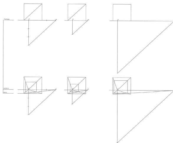
Profondeur et point de distance
